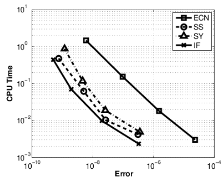
(b) ETD-CN
